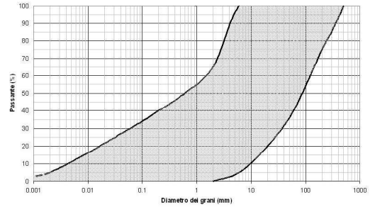
FUSO GRANULOMETRICO INDICATIVO
