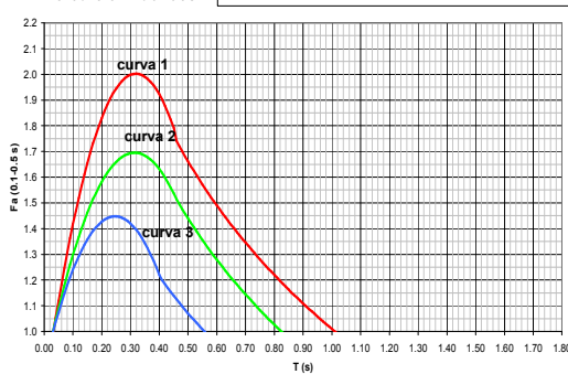
Correlazione T - Fa (0.1-0.5 s)
