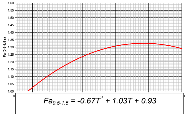
Correlazione T - Fa 0.5-1.5 s
