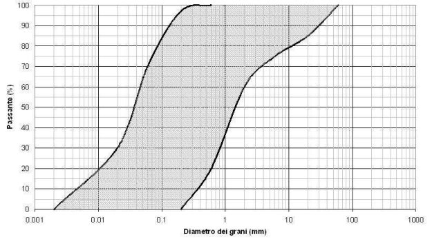
FUSO GRANULOMETRICO INDICATIVO
